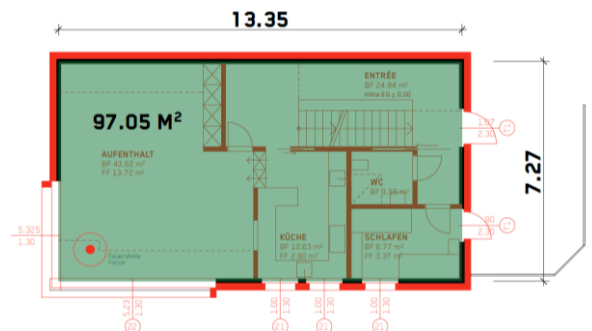
Erdgeschoss mit Aufenthaltsraum links, Entrée, Küche, sowie WC EG mit Dusche und Leiterschlafräum mit 6 Betten auf 3 Etagen rechts
